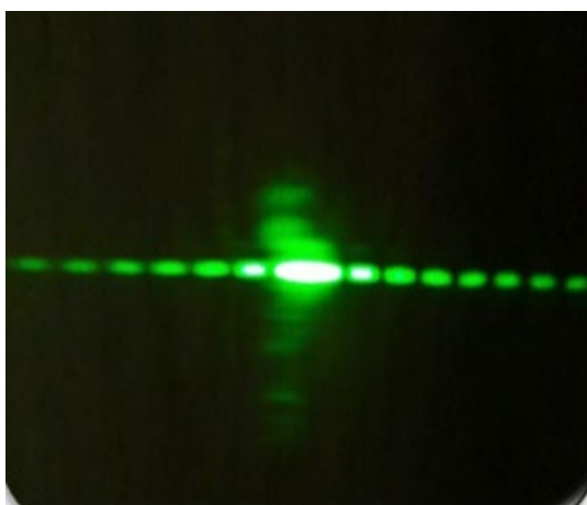
Figura 11- Difração em Fio
