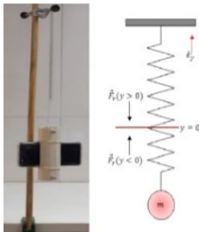
Figura 5 – Aparato experimental do MHA.
