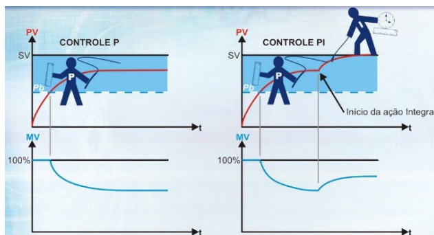
Figura 5 – Atuação de um Controlador P e PI.
