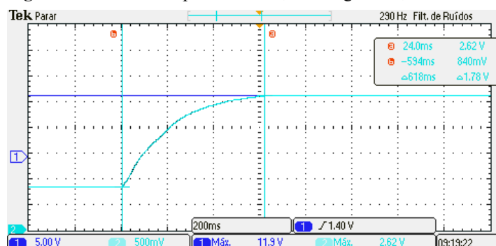
Figura 14 – Ganho Proporcional = 3,0 e Integral = 0,3.
