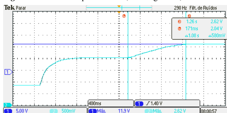
Figura 12 – Ganho Proporcional = 3,0 e Integral = 0,35.
