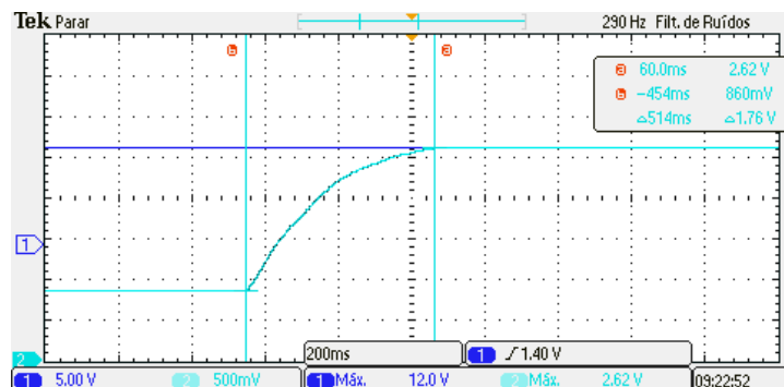
Figura 15 – Ganho Proporcional = 3,0 e Integral = 0,35.
