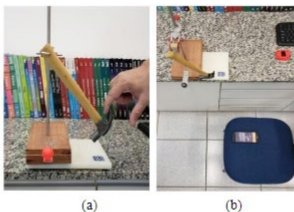
Figura 11 – Em (a) aparato experimental para coleta de intervalos de tempo e cálculo da aceleração gravitacional local. Em (b) cronômetro acústico do Phyphox coletando o tempo de queda da esfera.
