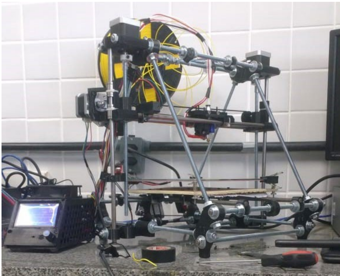
Figura 4: Impressora 3D modelo Prusa Mendel IT2 modificada.
