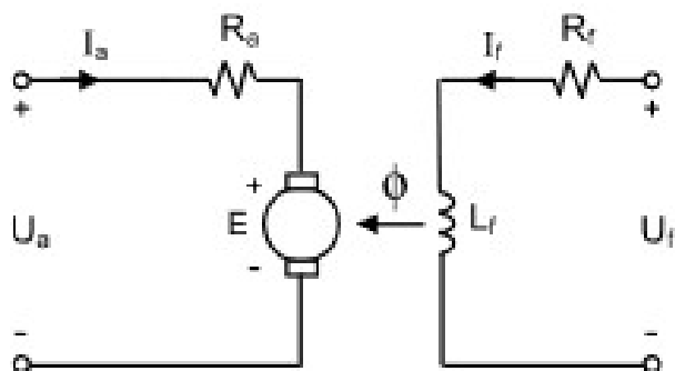
Figura 2 – Esquemático Motor CC independente de imã permanente.
