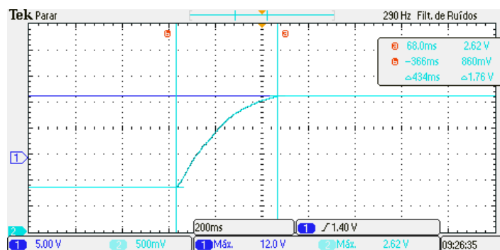
Figura 16 – Ganho Proporcional = 3,0 e Integral = 0,4.
