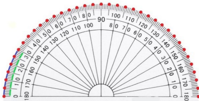
Figura 7 – Exemplo de Interpolação Linear.
