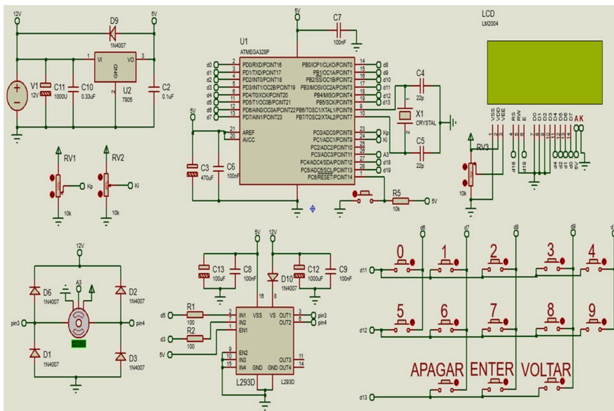
Figura 1 – Esquemático do circuito elaborado.
