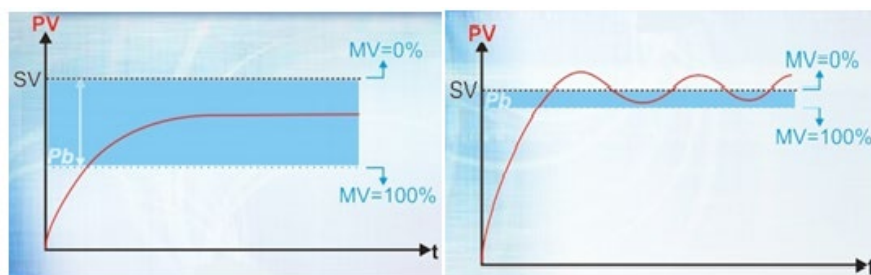
Figura 4 – Atuação de um Controlador Proporcional.
