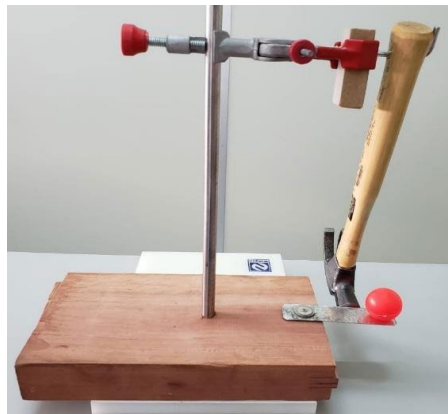
Figura 10 – Aparato experimental para abandono da esfera que entrará em queda livre.
