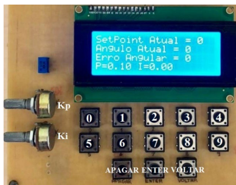
Figura 10 – Interface do kit didático desenvolvido.
