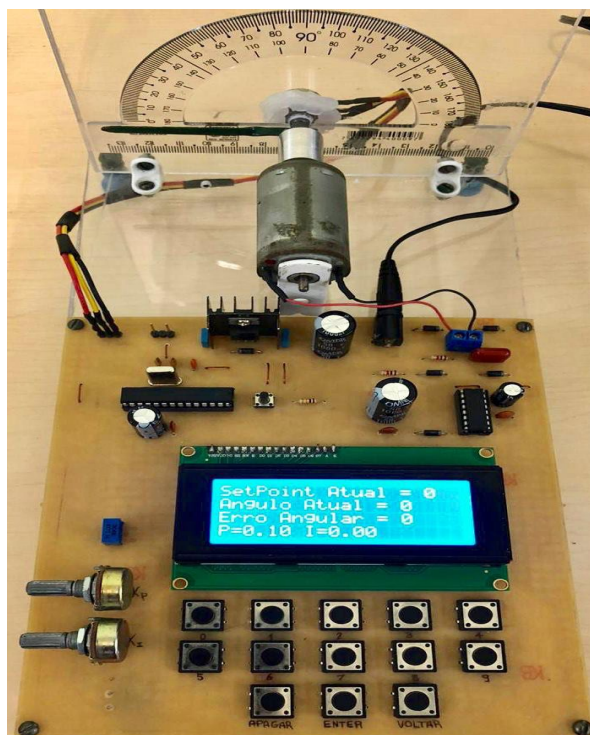
Figura 9 – Kit didático desenvolvido.
