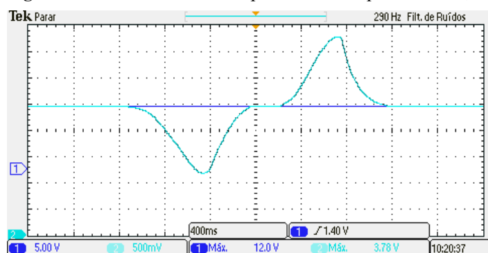
Figura 17 – Distúrbios externos para Ganho Proporcional = 3,0 e Integral = 0,25.
