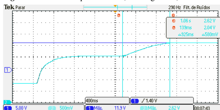
Figura 13 – Ganho Proporcional = 3,0 e Integral = 0,4.
