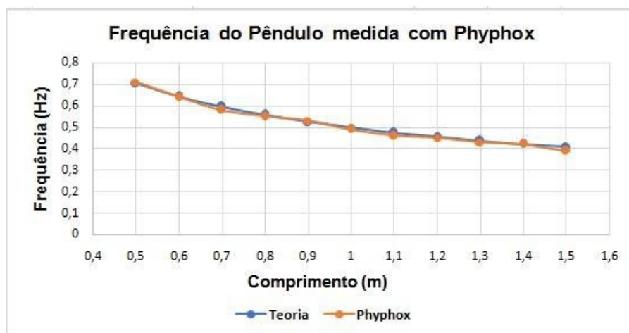
Figura 4 – Comparativo entre dados da teoria e do experimento Pêndulo com auxílio do Phyphox .
