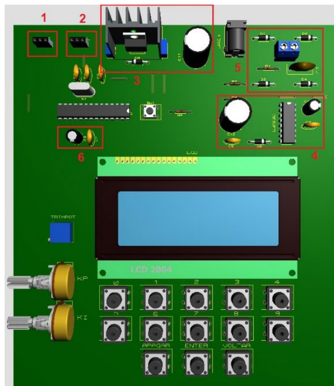
Figura 8 – Visualização 3D da placa de circuito impresso projetada.
