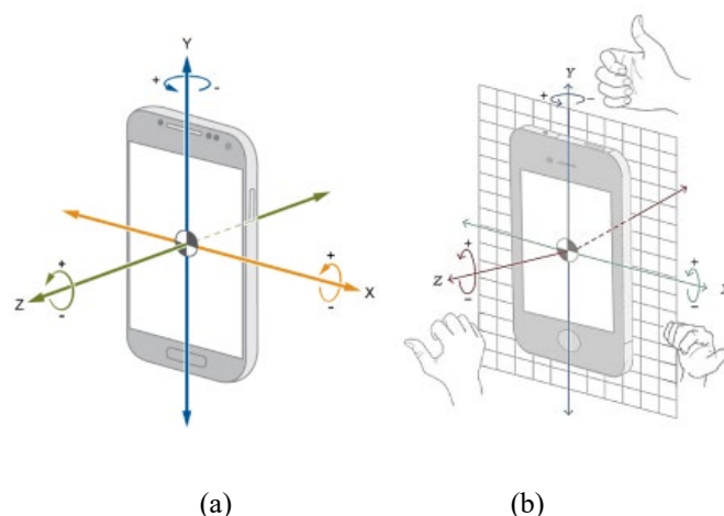
Figura 1 – Em (a) eixos cartesianos para análise dos movimentos de rotação do Smartphone e em (b) espaço euclidiano para análise da sua translação.
