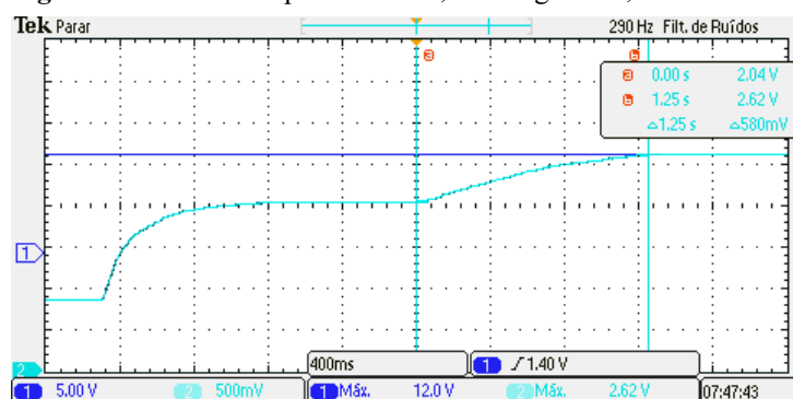
Figura 11 – Ganho Proporcional = 3,0 e Integral = 0,3.
