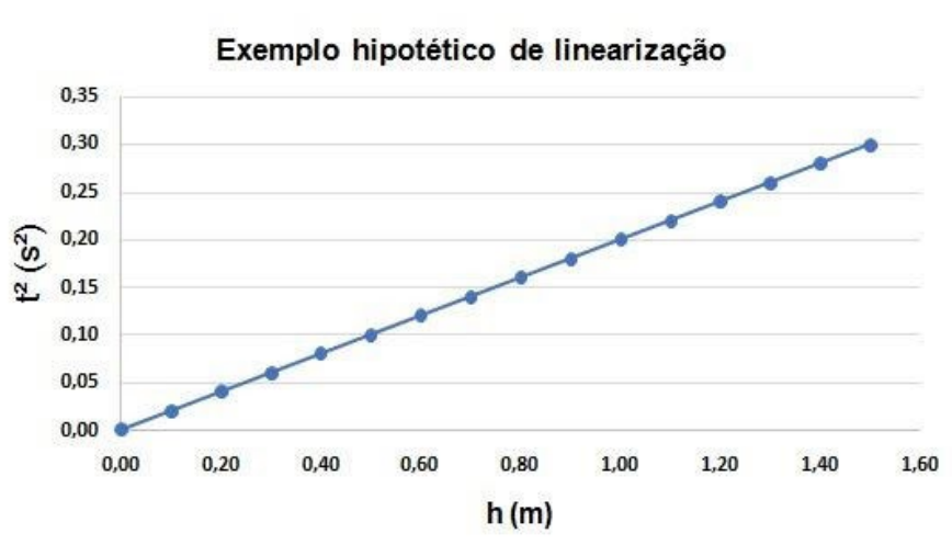
Figura 9 – Exemplo de linearização de uma função de grau 2.
