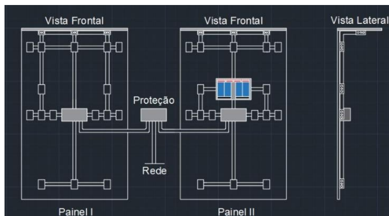
Figura 1. Esquemático dos painéis de instalações elétricas
